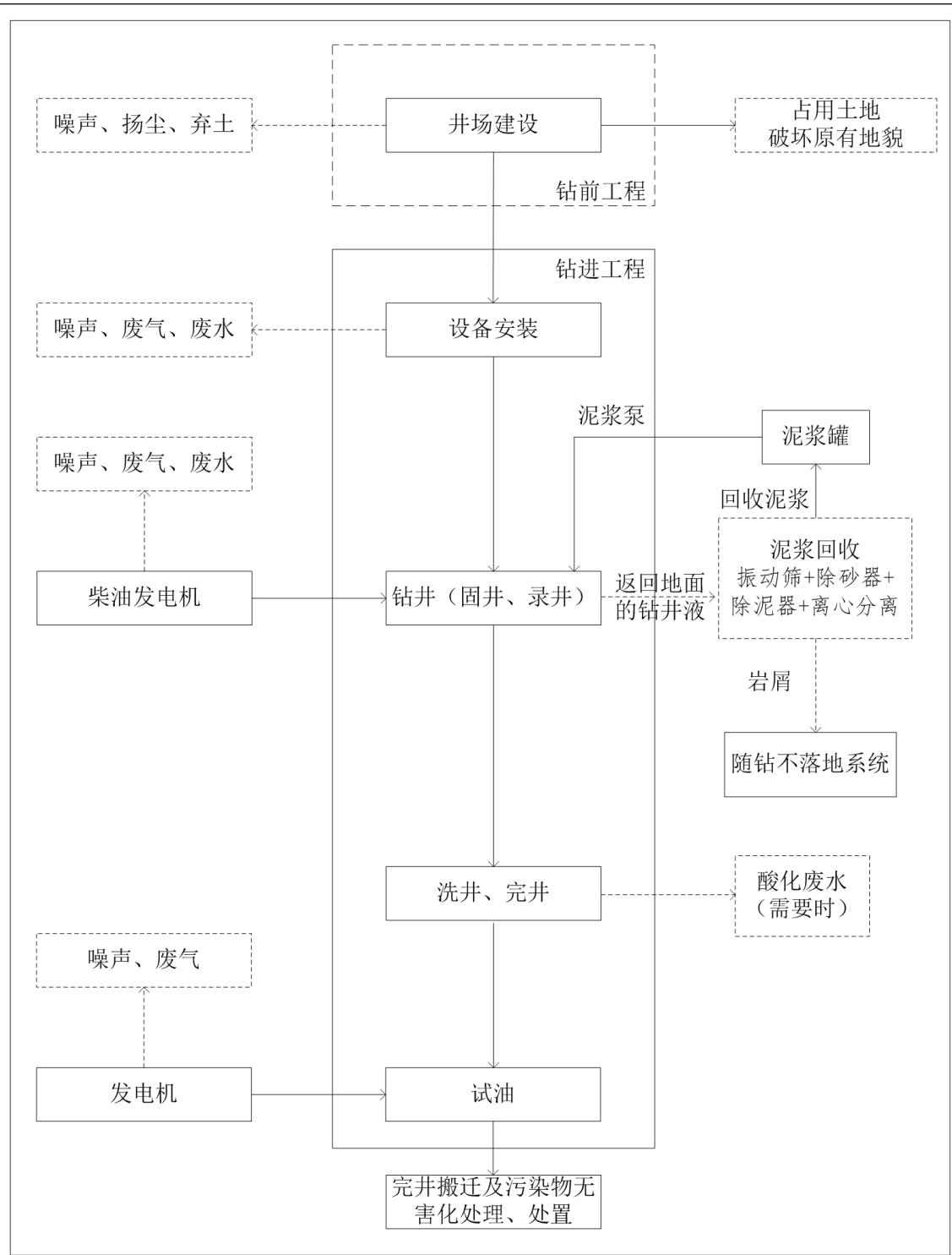
图 2-6 钻井工艺流程及产污环节示意图
