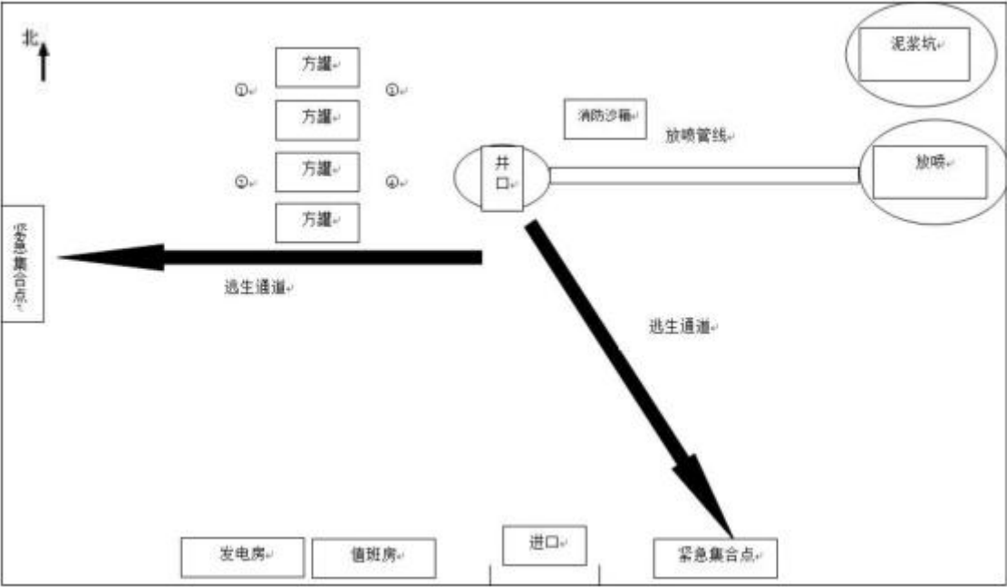
图 2-4 试油井场平面布置示意图
