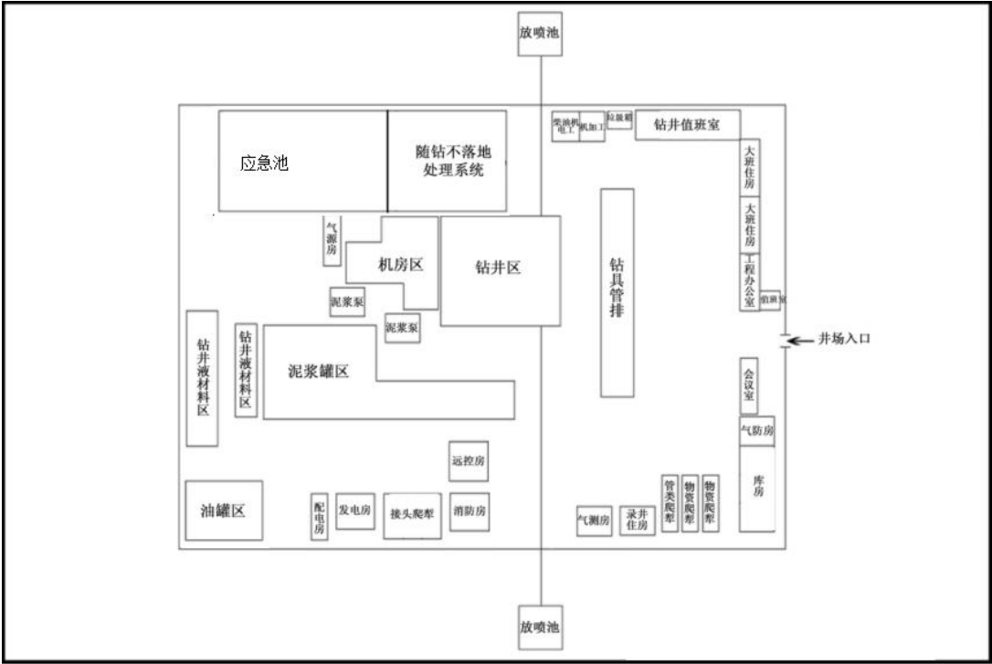
图 2-3 钻井井场平面布置示意图
